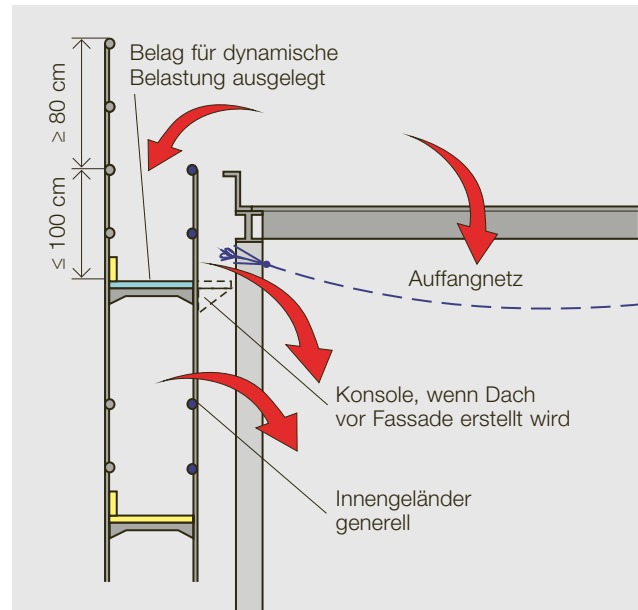
Bild 23: Montagebau
