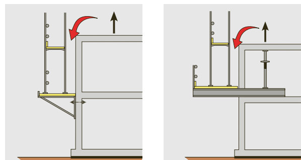
Bild 7: Konsolgerüst
