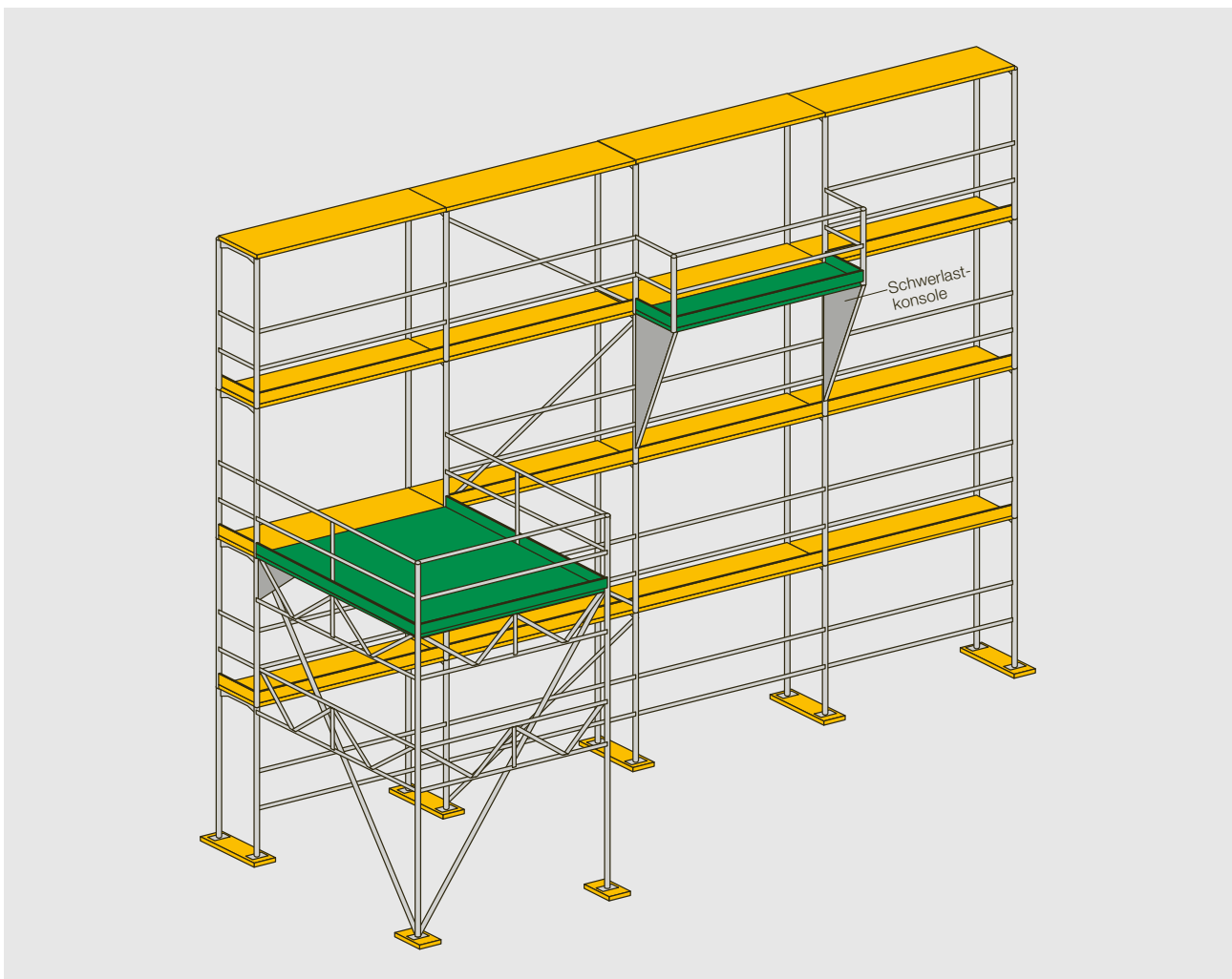
Bild 25: Versetzte Podeste für den Materialumschlag
