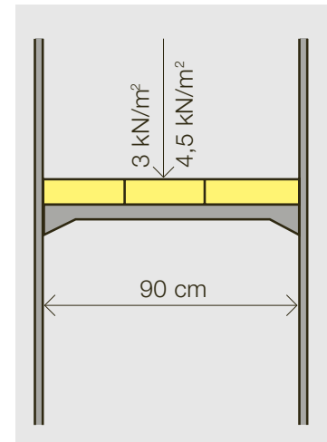
Bild 3: Maurergerüst bzw. Steinhauergerüst
